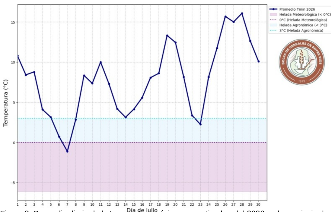
Figura 2: Promedio diario de la temperatura mínima en septiembre del 2026 en la provincia de Entre Ríos.
