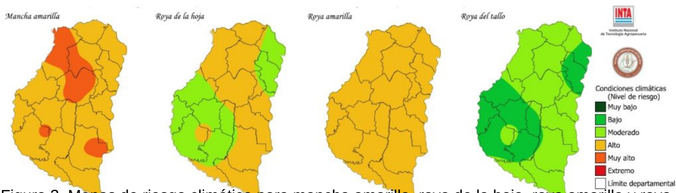
Figura 3. Mapas de riesgo climático para mancha amarilla, roya de la hoja, roya amarilla y roya del tallo en la provincia de Entre Ríos, correspondientes al período comprendido entre el 30 de septiembre y el 6 de octubre de 2026.
