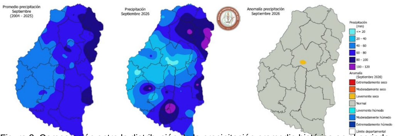
Figura 2: Comparación entre la distribución de la precipitación promedio histórica en el periodo (2004 – 2025), septiembre del 2026 y la anomalía resultante.
