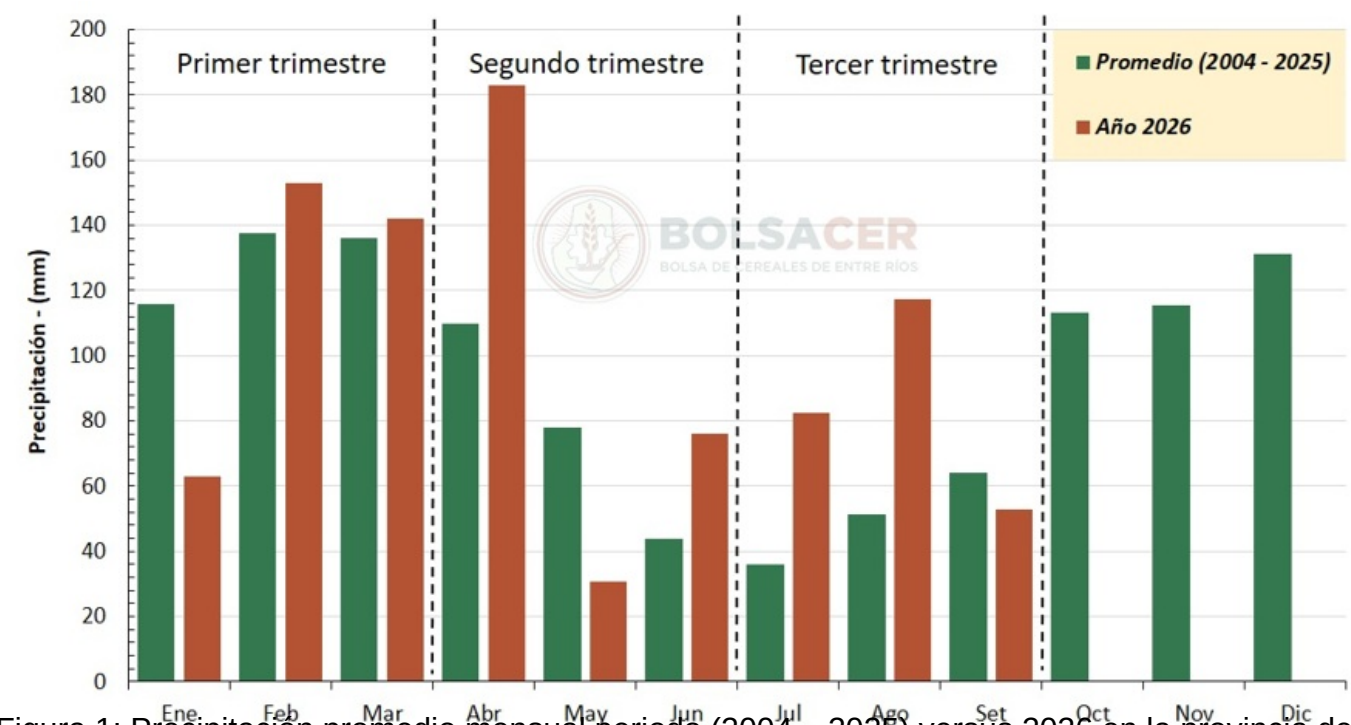
Figura 1: Precipitación promedio mensual periodo (2004 – 2025) versus 2026 en la provincia de
